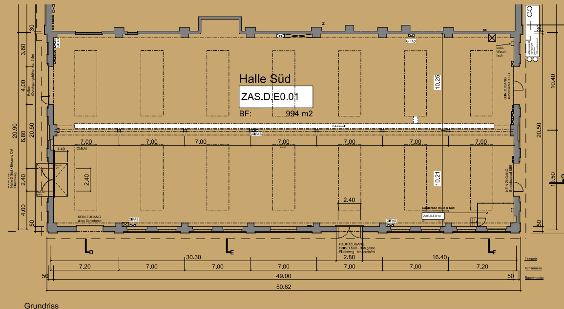
Grundriss
