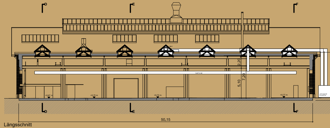
Längsschnitt
