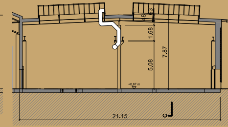
Querschnitt
